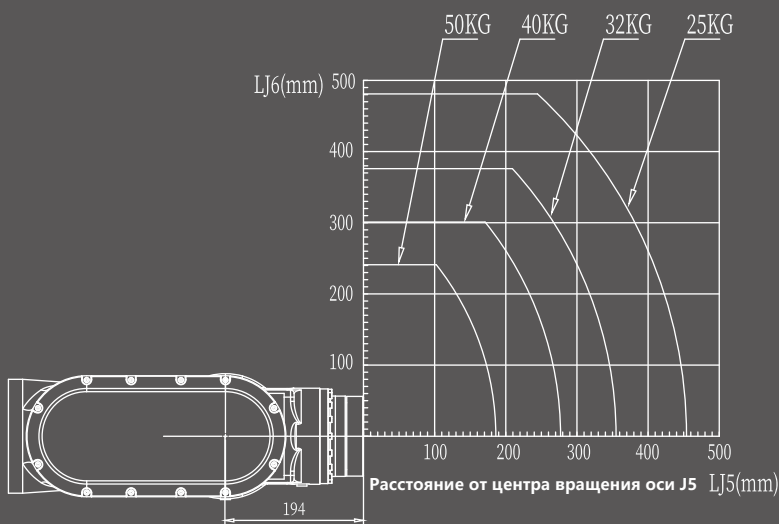
Диаграмма кривой диапазона нагрузки SF50 - C2185
